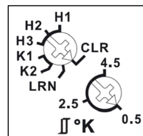
Funksjonsvelgere (Fabrikkinnstilling)
